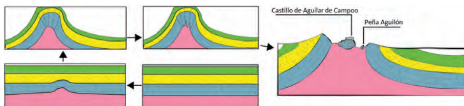
Figura 4. Evolución del anticlinal diapírico de Aguilar de Campoo. Fuente: Elaboración de los autores.
